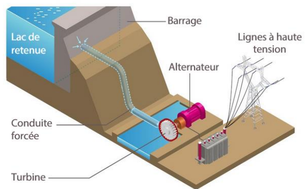
La centrale hydroélectrique
